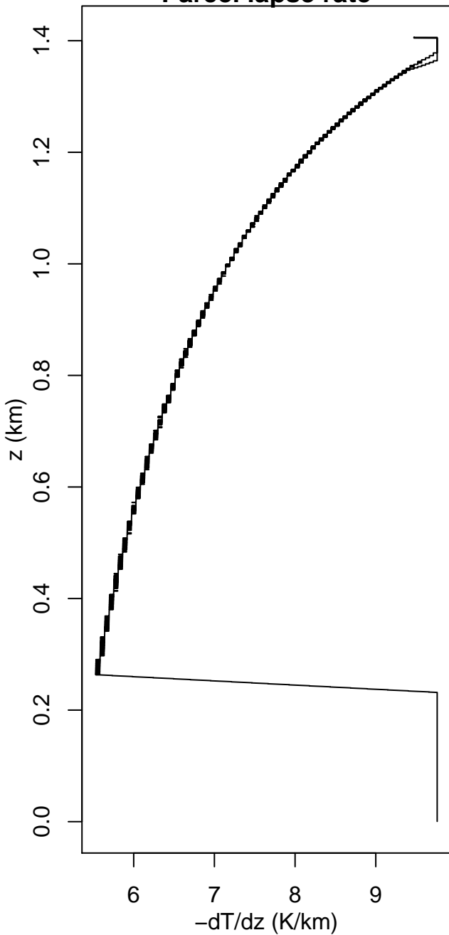
Parcel lapse rate
